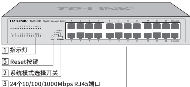
图1-5 TL-SG2024D前面板示意图
